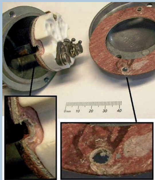
Bild 6 Weichasbestzeugnis „Kautasit“ als Dichtungsmaterial für wassertechnische Anlagen und für Rohrleitungsflansche [C.1]
