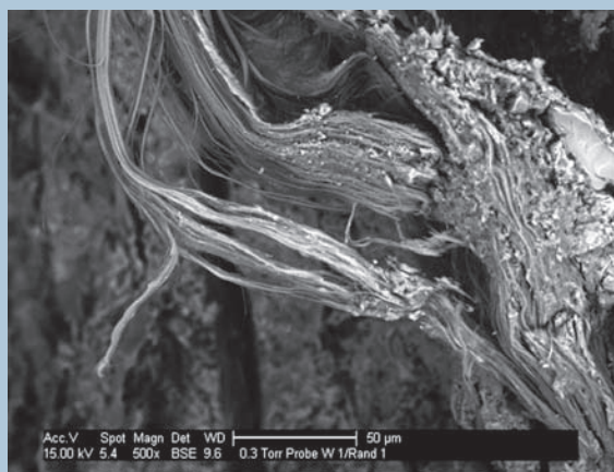
Bild 9 ESEM-REM-Aufnahme von stark gebundenen Asbestfasern in der Bruchfläche einer zementgebundenen Kunstschieferplatte [C.4]
